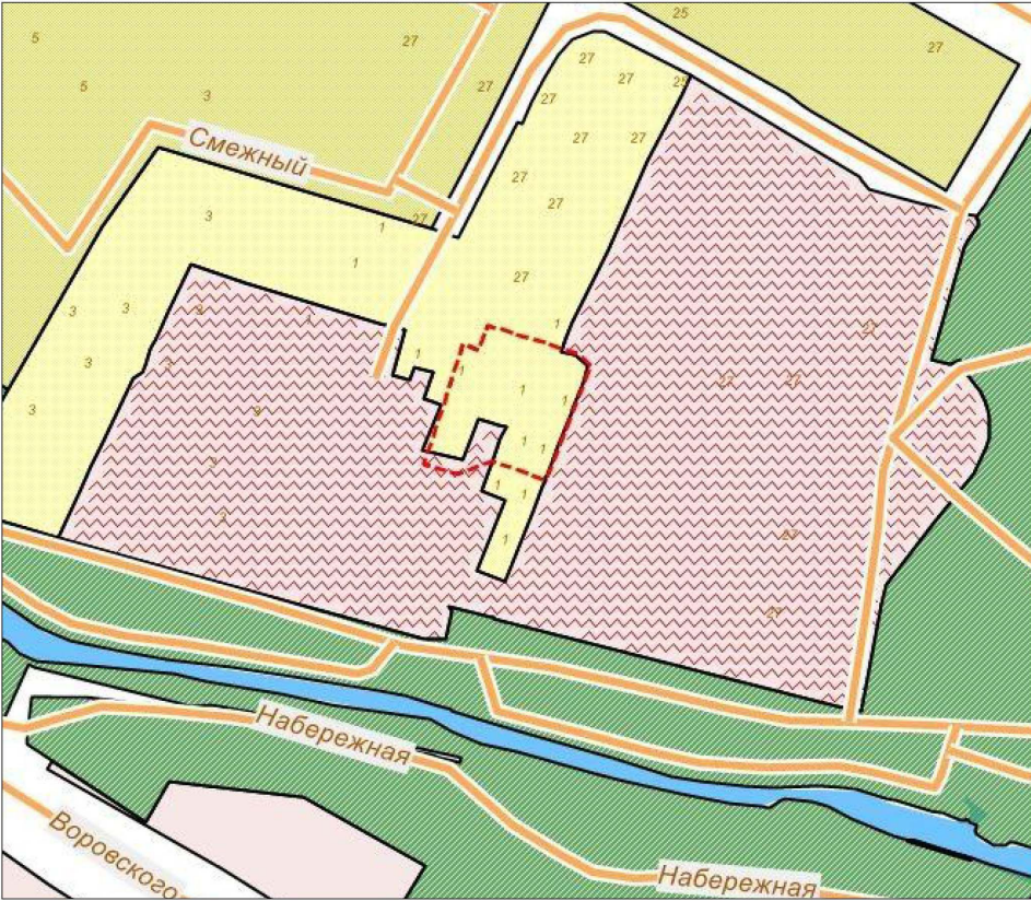
Схема градостроительного зонирования до внесения изменений для земельного участка, расположенного по адресу: Республика Крым, г. Симферополь, ул. Гаспринского, 3
