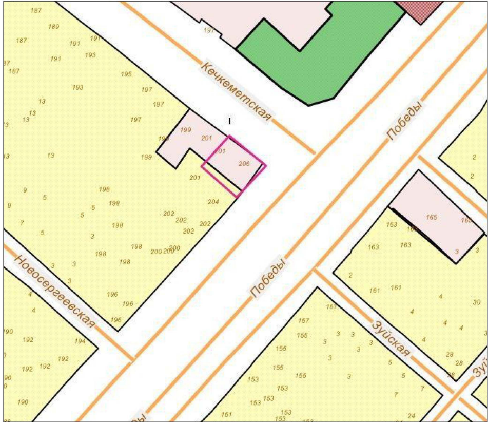
Схема градостроительного зонирования до внесения изменений для земельного участка, расположенного по адресу: Республика Крым, г. Симферополь, улица Кечкеметская, земельный участок 206/203, с кадастровым номером 90:22:010204:1146
