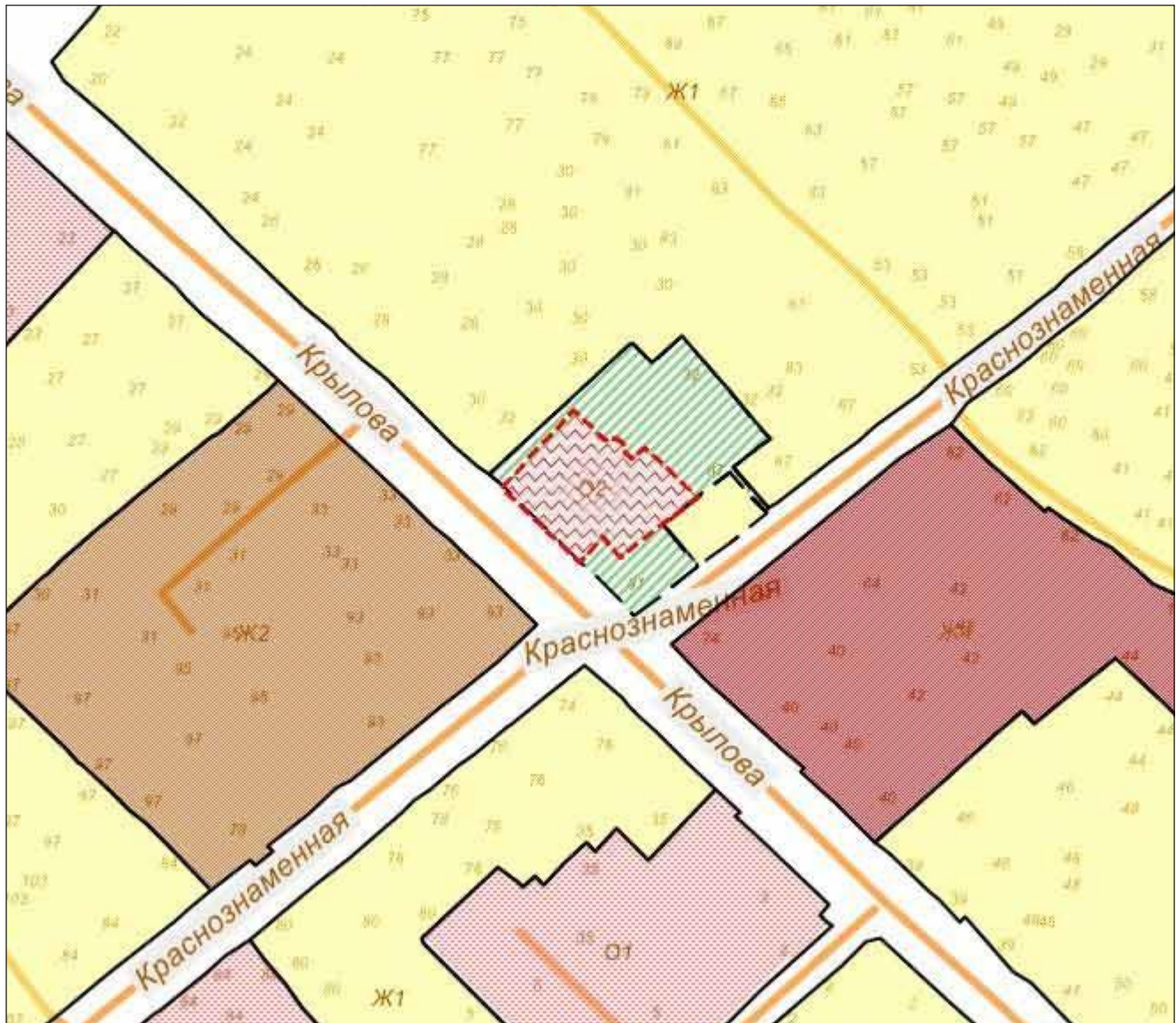
Схема градостроительного зонирования после внесения изменений для земельного участка по адресу: Республика Крым, г. Симферополь, ул. Крылова, д. 32а, с кадастровым номером 90:22:010303:4789
