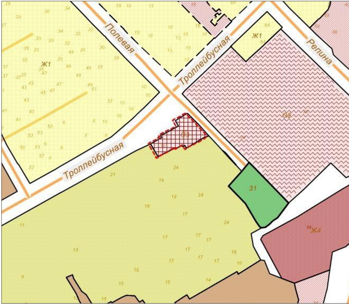
Схема градостроительного зонирования до внесения изменений для земельного участка по адресу: Республика Крым, г. Симферополь, ул. Полевая/ул. Троллейбусная, 24/23, с кадастровым номером 90:22:010217:4095
