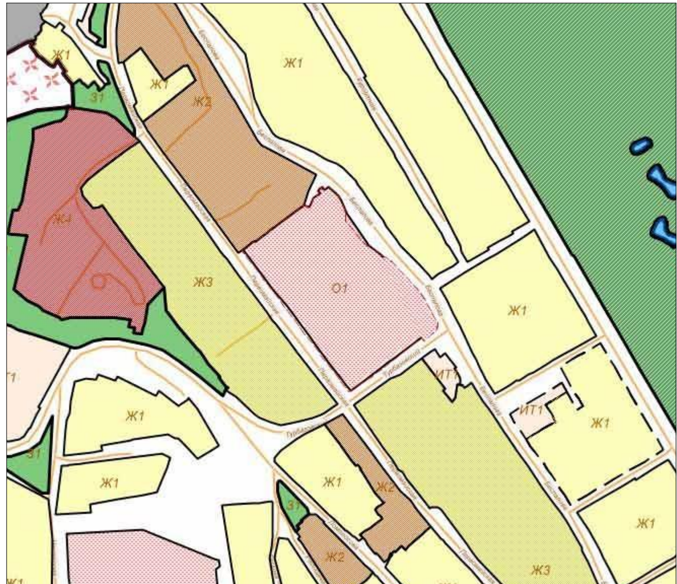
Схема градостроительного зонирования после внесения изменений для земельного участка по адресу: Республика Крым, г. Симферополь, ул. Беспалова, уч. 21, с кадастровым номером 90:22:010225:6610
