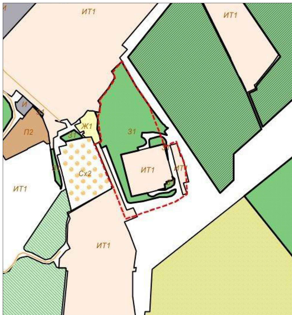
Схема градостроительного зонирования до внесения изменений для земельного участка по адресу: Республика Крым, г. Симферополь, в районе ул. Балаклавской
