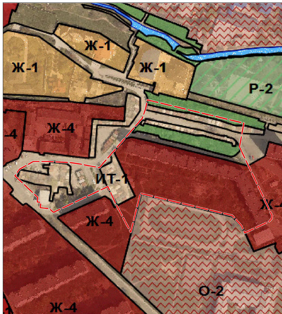
Схема градостроительного зонирования до внесения изменений для земельного участка по адресу: Республика Крым, г.Симферополь, ул.Лермонтова, 35
