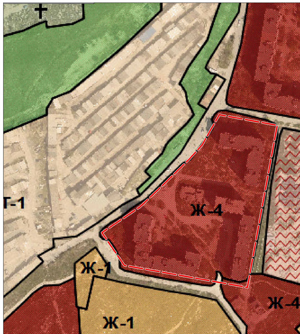
Схема градостроительного зонирования до внесения изменений для земельного участка по адресу: Республика Крым, город Симферополь, ул.Ковыльная,36.
