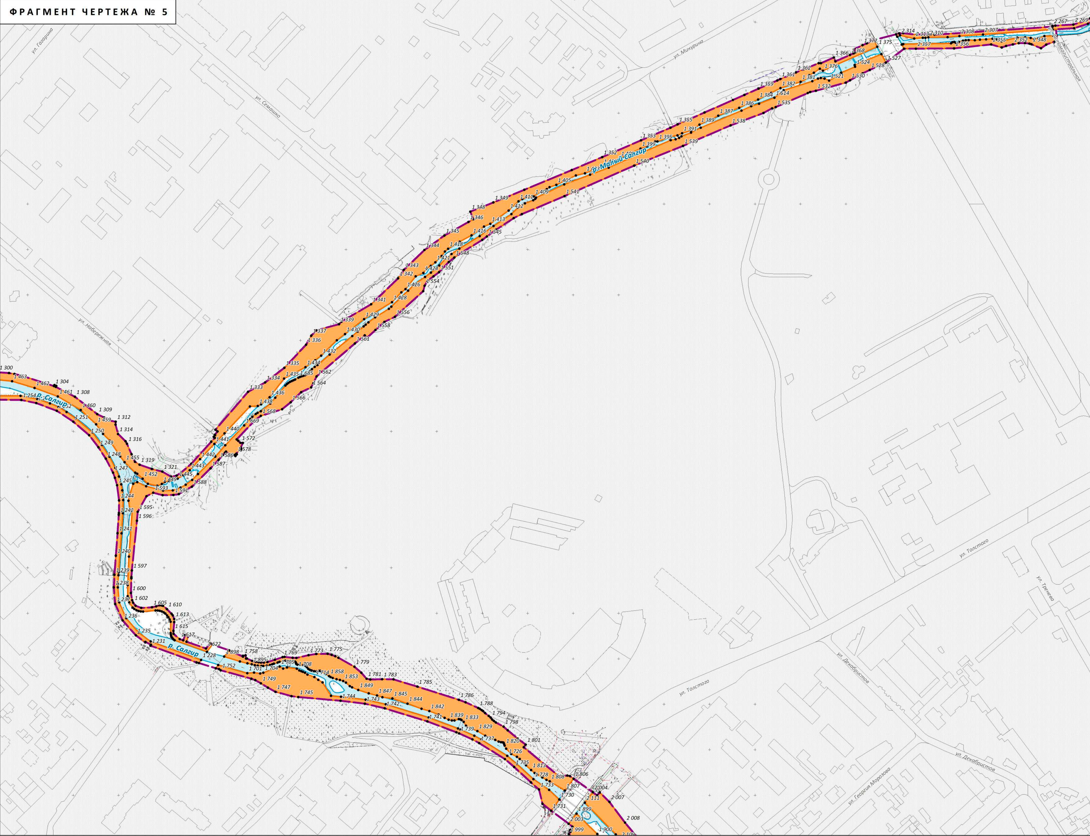
ФРАГМЕНТ ЧЕРТЕЖА № 5
