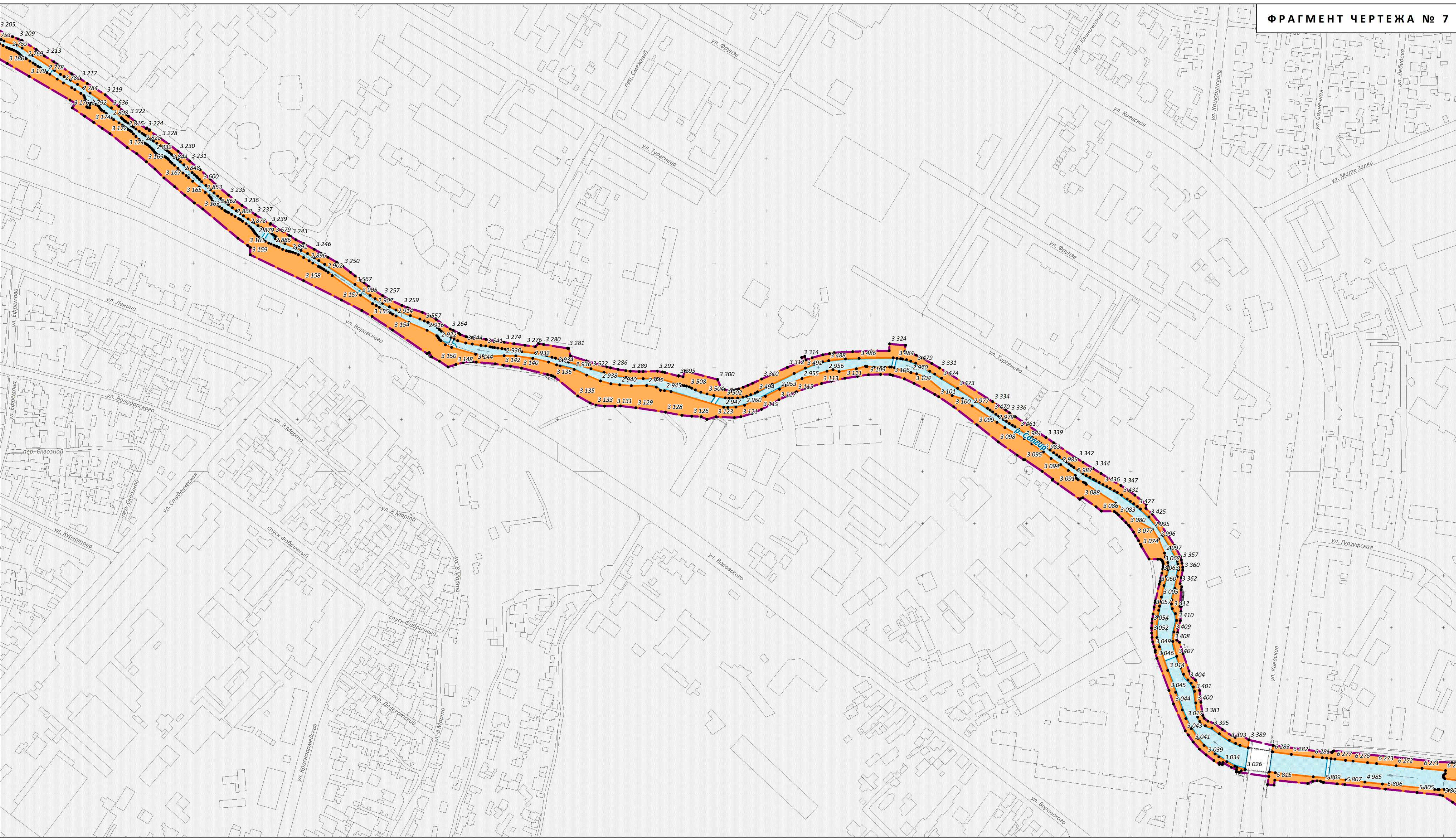
ФРАГМЕНТ ЧЕРТЕЖА № 7
